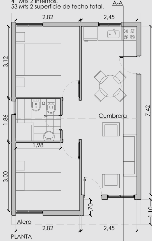
PLANTA
